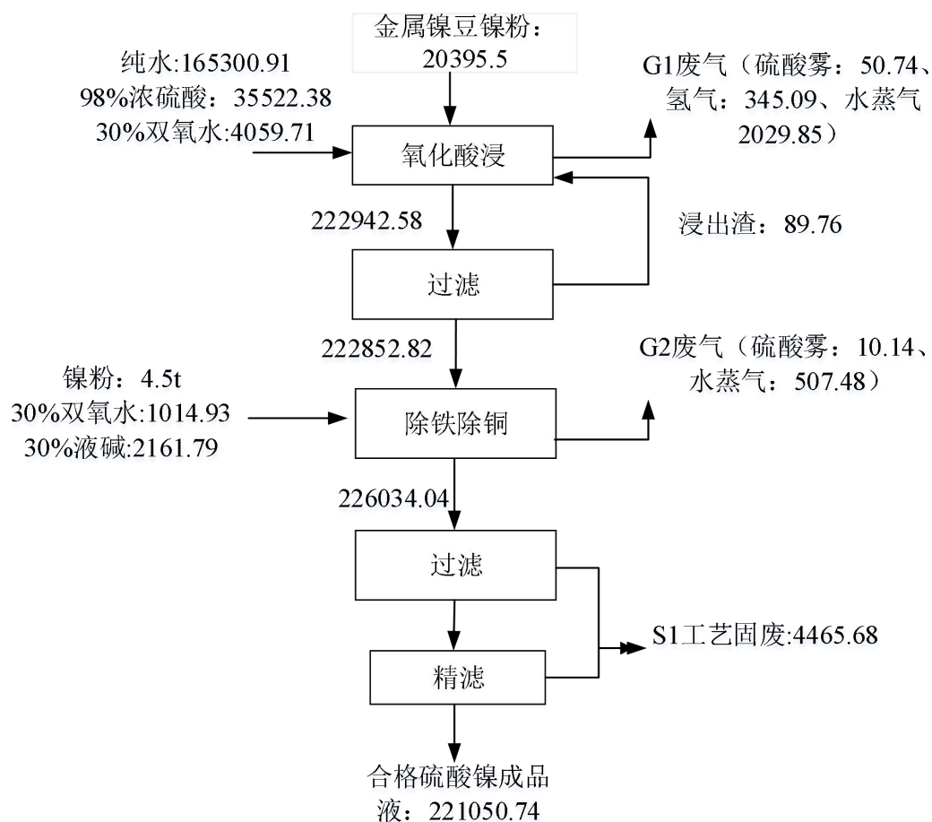
图 5.2-1 镍豆镍粉溶解生产车间物料平衡图 （单位：t/a）
