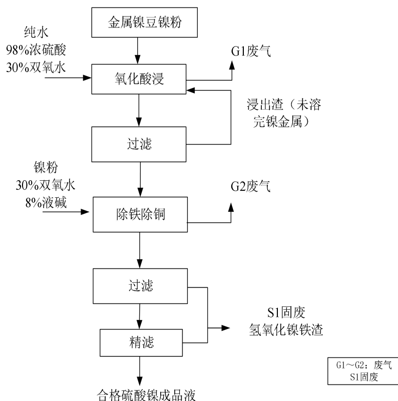
图 3.6-1 镍豆镍粉制硫酸镍成品液工艺流程及产污环节图
