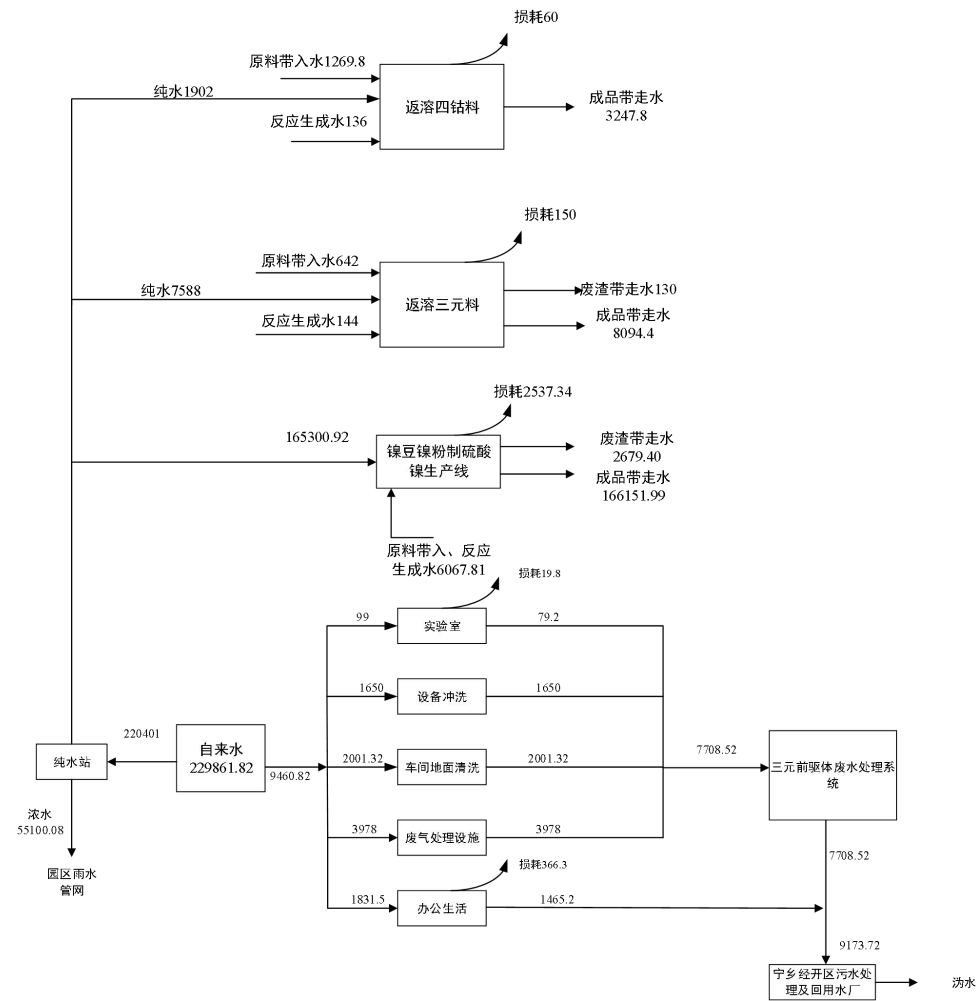
图 5.2-3 扩建后四期工程运营期水平衡图单位： \text{m}^3/\text{a}
