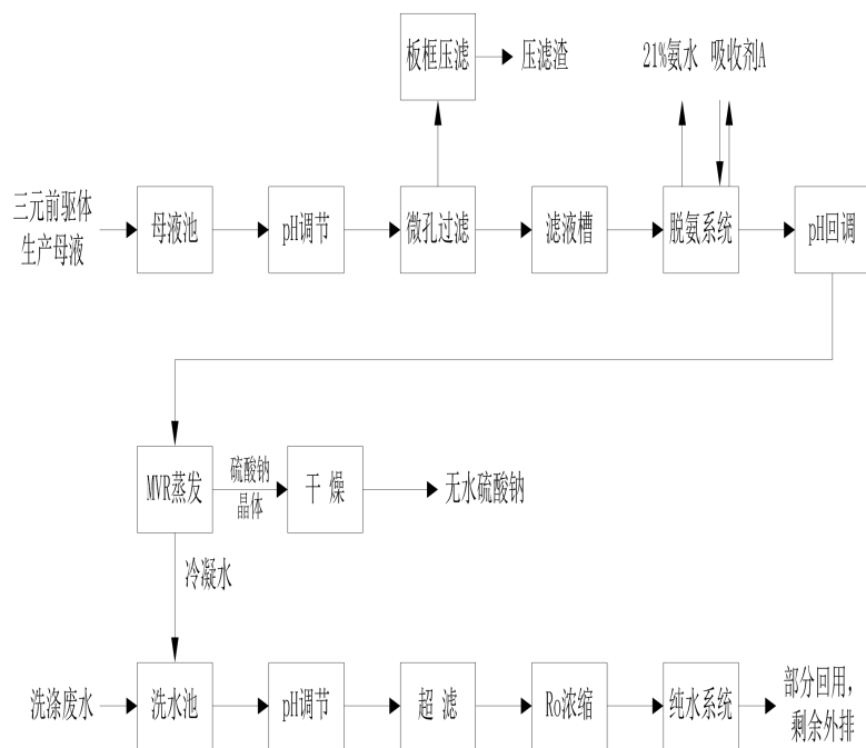
图 3.6-2 三元返溶料制三元溶液工艺流程及产污环节图
