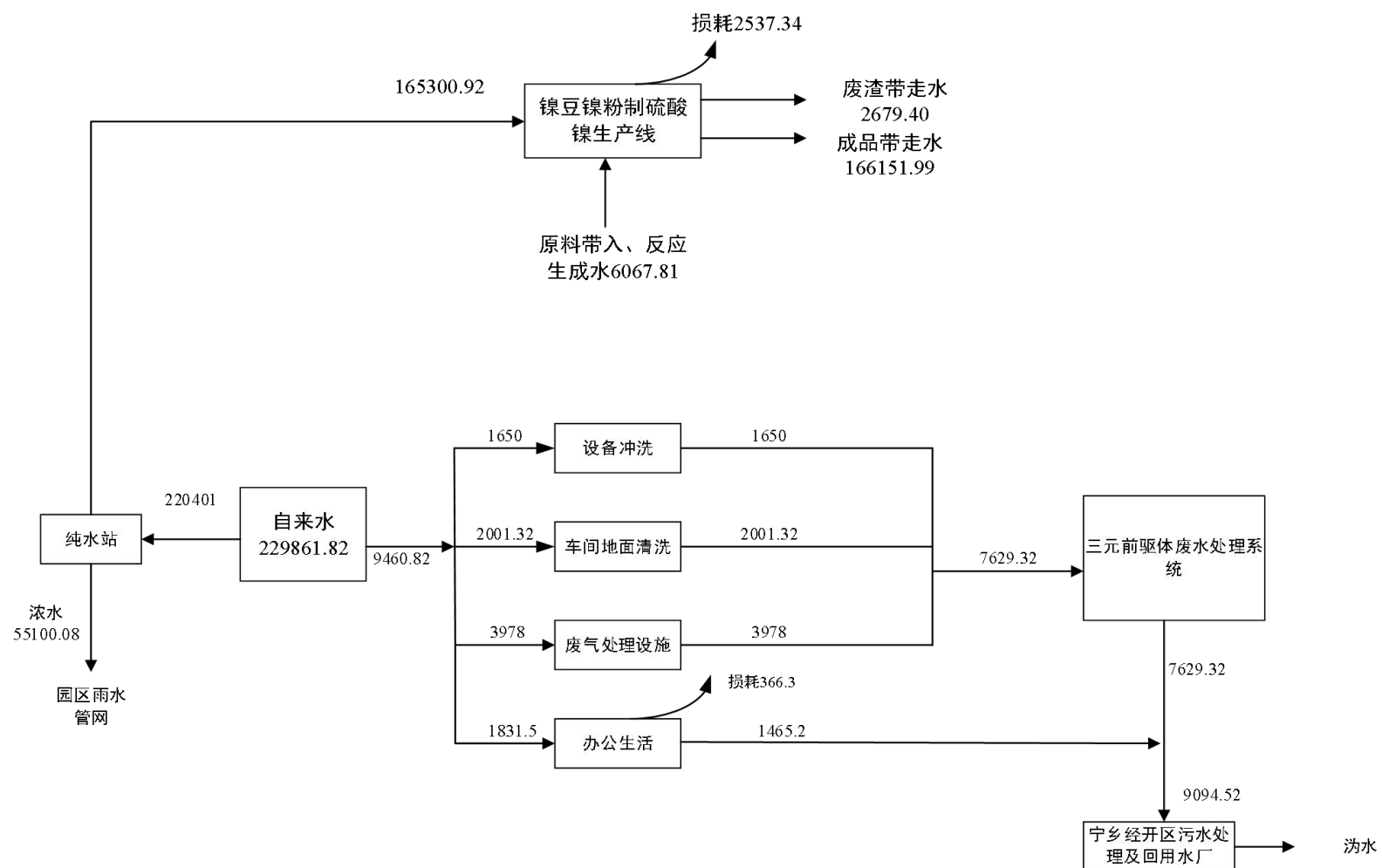
图 5.2-2 本项目运营期水平衡图单位：m³/a
