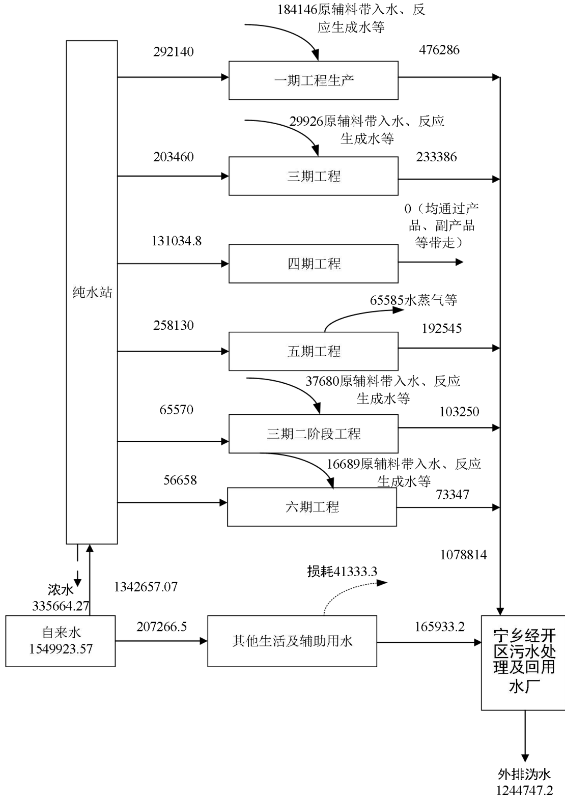
图 5.2-4 扩建后全厂运营期水平衡图 单位: \text{m}^3/\text{a}
