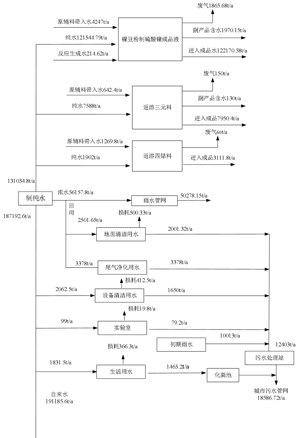
图 3.7-1 四期工程水平衡图
