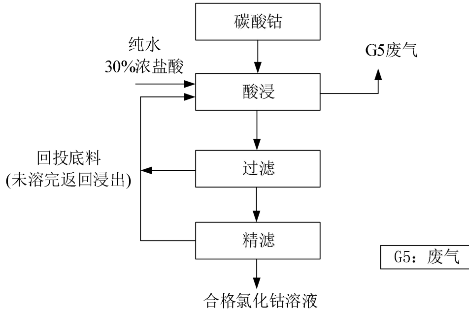
图 3.6-3 四钴料加工工艺流程及产污环节图
